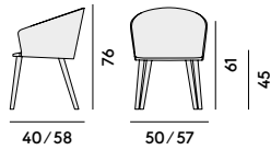
047 Poltroncina con struttura in acciaio/ Armchair with steel frame
