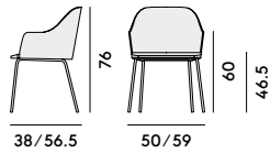
025 Poltroncina con struttura in acciaio e sedile imbottito / Armchair with steel frame and upholstered seat
