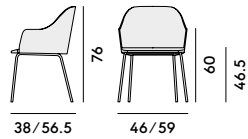
032 Poltroncina con struttura in acciaio, imbottita / Armchair with steel frame, upholstered
