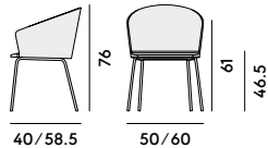
051 Poltroncina con struttura in acciaio e sedile imbottito / Armchair with steel frame and upholstered seat
