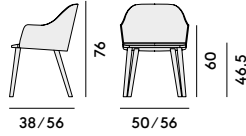
023 Poltroncina con struttura in acciaio e sedile imbottito / Armchair with steel frame and upholstered seat
