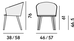
049 Poltroncina con struttura in acciaio, imbottita / Armchair with steel frame, upholstered
