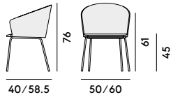
050 Poltroncina con struttura in acciaio/ Armchair with steel frame
