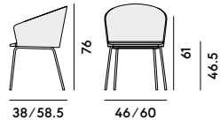
052 Poltroncina con struttura in acciaio, imbottita / Armchair with steel frame, upholstered
