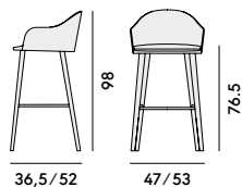
028 Sgabello in frassino, con sedile imbottito / Barstool in ashwood, with upholstered seat
