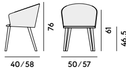
048 Poltroncina con struttura in acciaio e sedile imbottito / Armchair with steel frame and upholstered seat
