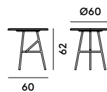
722 Tavolo con struttura in acciaio e piano in frassino / Table with steel frame and top in ashwood
